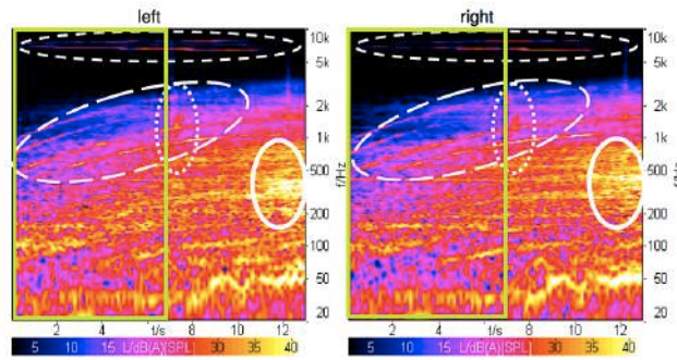
Figure 13 : Spectrogramme du bruit de fond intérieur lors d'une accélération de 0 à 50 km/h, [10].
