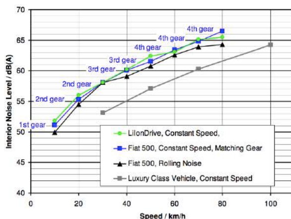
Figure 19 : Comparaison des niveaux perçus dans l'habitacle de différents véhicules à vitesse constante à différentes vitesses (Niveau = f[vitesse]), [11].
