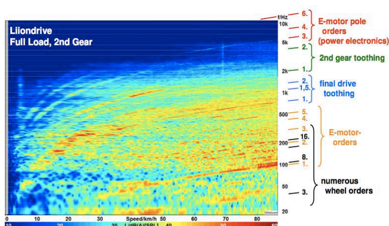
Figure 15. : Spectrogramme de l'habitacle de la Fiat 500 LiionDrive - Fréquence = f (vitesse), [11].
