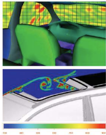
Figure 13 : Simulations d'écoulements d'air sur un véhicule à toit ouvrant ou sur les vitrages [8]
