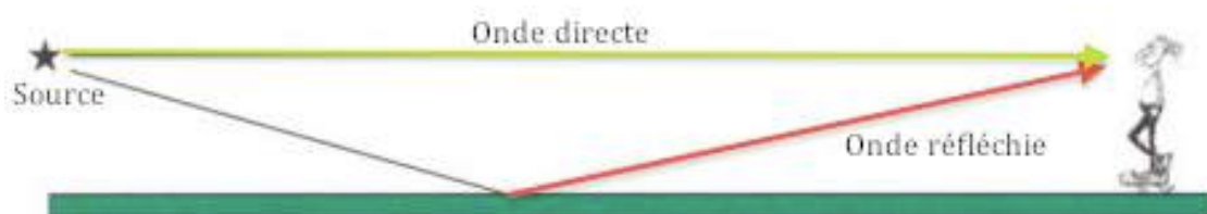
Figure 5 : Représentation du trajet de l'onde sonore, prenant en compte les effets de sol [Réf : acoustique environnementale BBRI.be]
