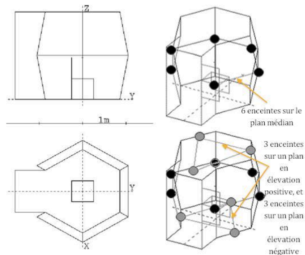
Figure 50 : Plan de l'installation permettant la restitution.
