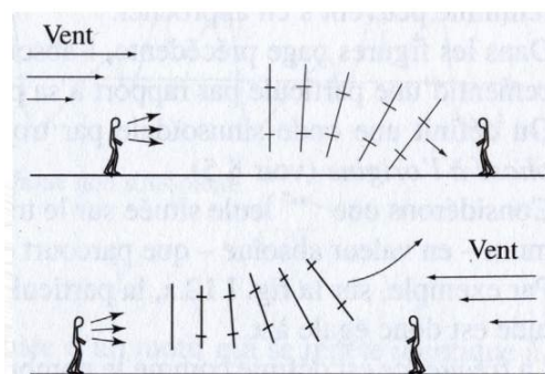
Figure 5 : Représentation du trajet des ondes sonores en fonction de leur position par rapport au vent [3]
