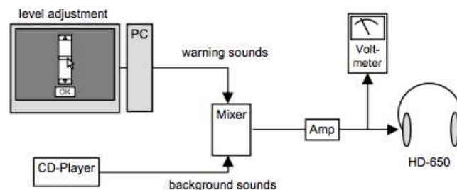
Figure 7 : Installation mise en place pour l'expérience.
