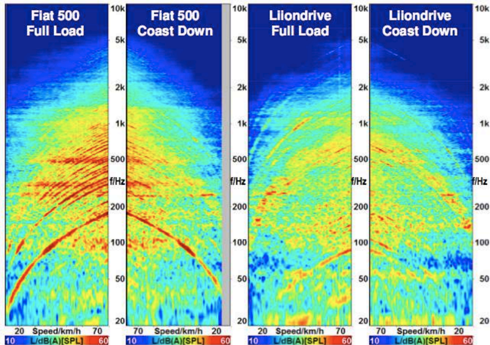
Figure 18 : Comparaison de l'acoustique de l'habitacle entre une Fiat 500 série et une Fiat 500 LiionDrive en phase d'accélération et de roue libre, [11].
