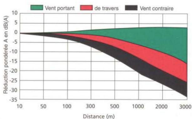
Figure 4 : Influence du vent sur la réduction du niveau sonore en fonction de la distance [3]
