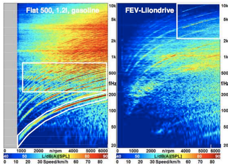
Figure 16 : Comparaison fréquentielle entre le moteur essence 1,2L 4 cylindres et du moteur tout électrique ( fréquence = f [tours/minutes] ), [11].
