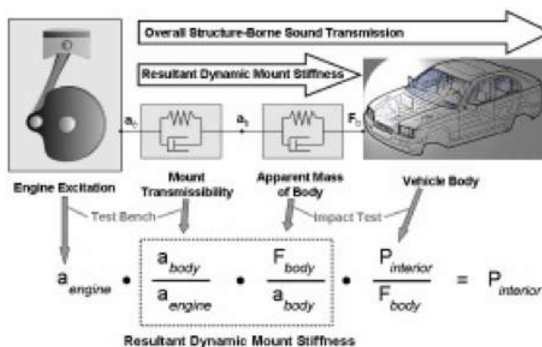
Figure 12 : Principe de mesure de transmission de bruit solidien dans l'habitacle selon la méthode VINS.
