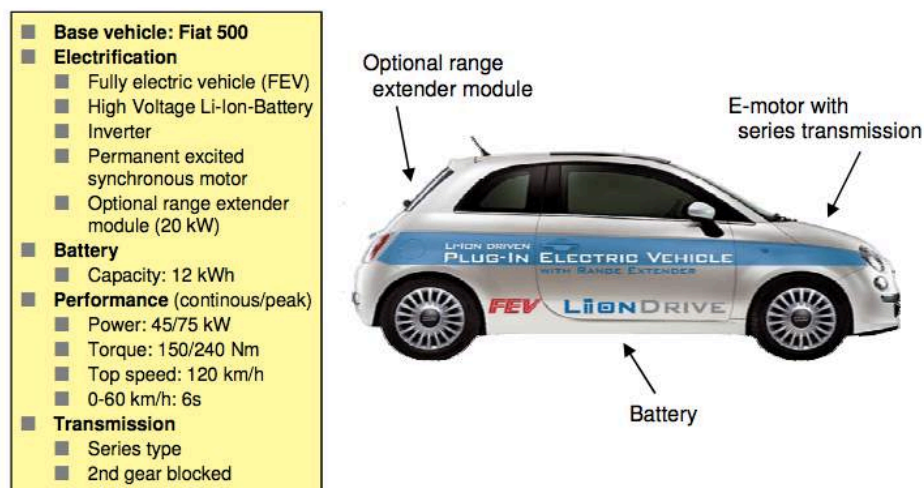
Figure 14 : Spécifications du prototype Fiat 500 LiionDrive, [11].
