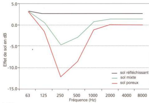
Figure 6 : Représentation de l'influence du sol sur l'atténuation (en dB) de certaines fréquences.
