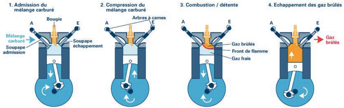
Figure 17 : Principe de fonctionnement d'un moteur thermique 4 cylindres
